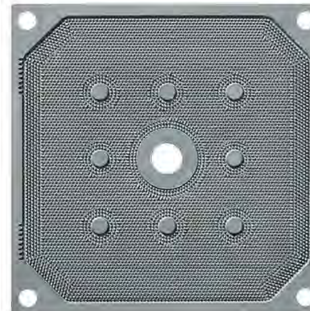
1250型隔膜滤板 1250 diaphragm filter plate
